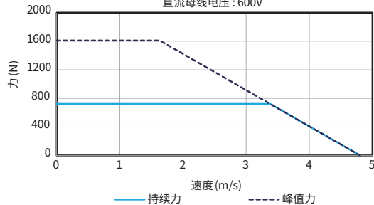
力速曲线 AKM100-B2 直流母线电压：600V
