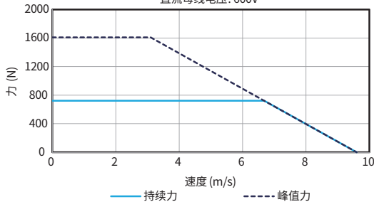
力速曲线 AKM50-B4 直流母线电压：600V
