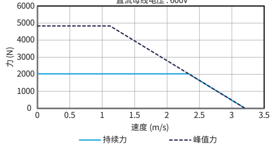
力速曲线 AKM150-B4 直流母线电压: 600V
