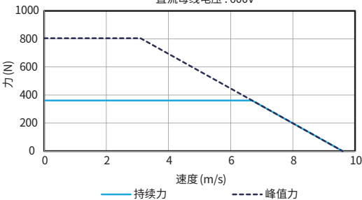
力速曲线 AKM50-B2 直流母线电压: 600V
