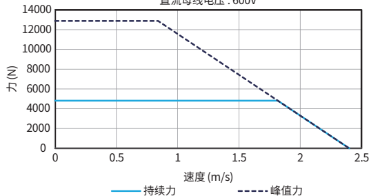
力速曲线 AKM200-B8 直流母线电压: 600V
